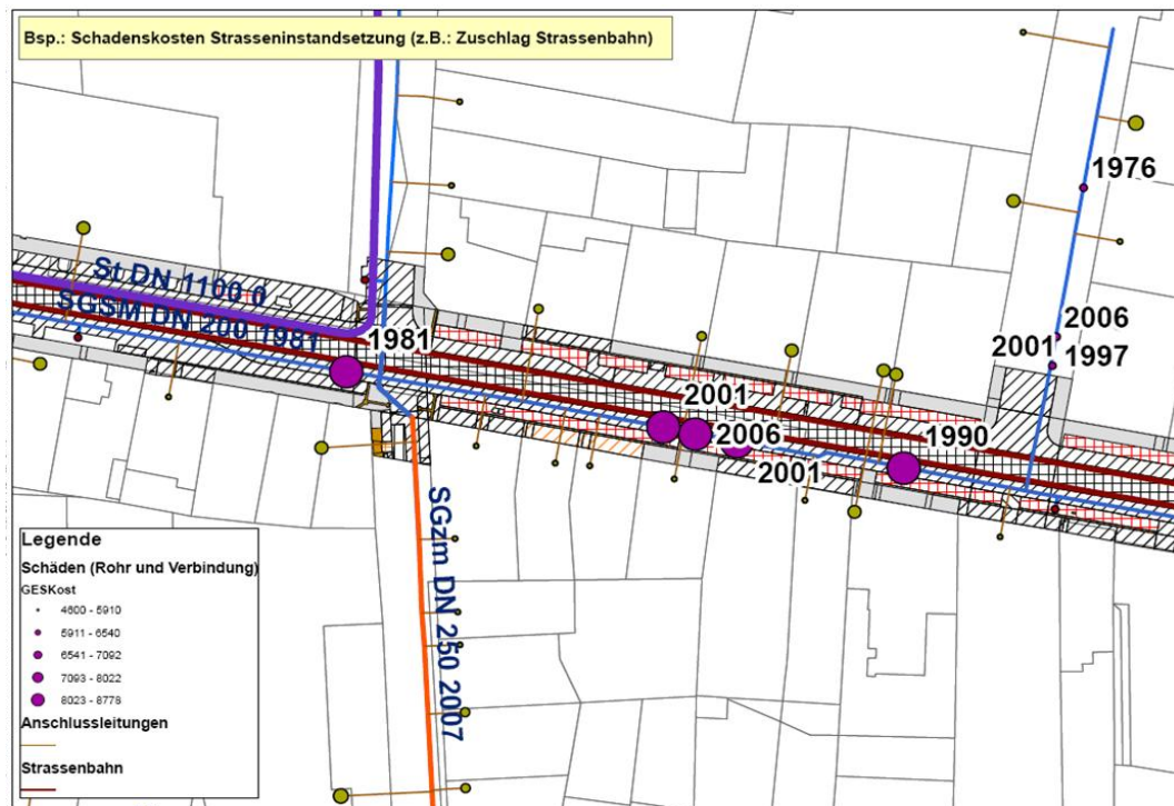
Abbildung 2: GIs gestützte Schadenskostenzuordnung in Abhängigkeit vom Strassenbelag und der Lage in der Straße
