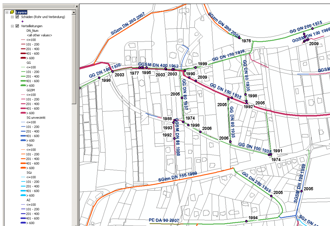
Abbildung 1: Leitungs- und Schadensdatenbasis GIS –gestützte Rehabilitationsplanung
