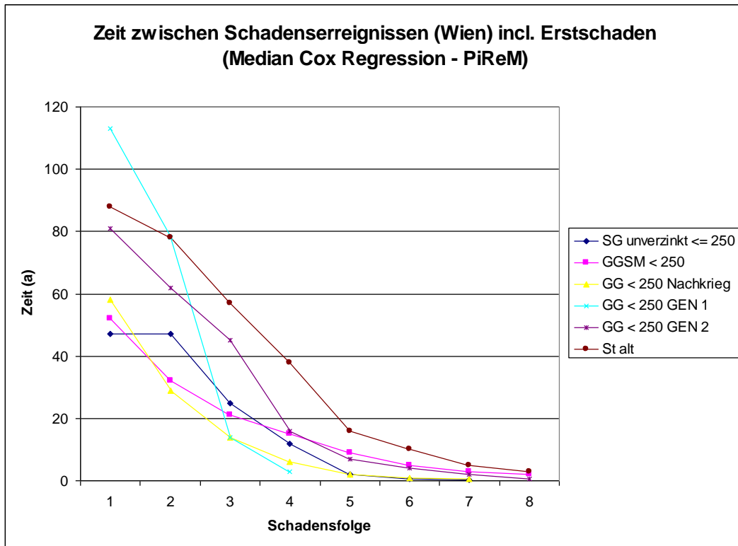
Abbildung 3: Medianwerte für Zeitabstände zwischen Leitungsschäden Wasserversorgungsleitungen Wien
